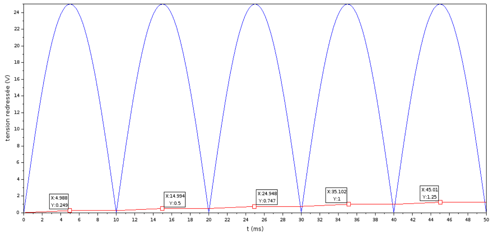
Charge des condensateurs de l'alimentation
