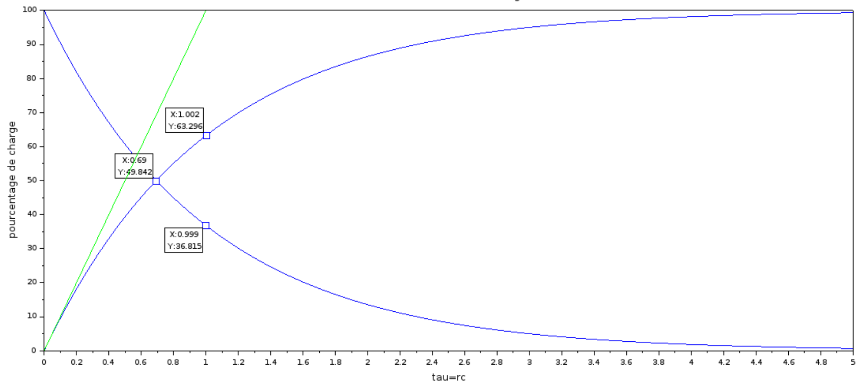
courbe universelle de charge
